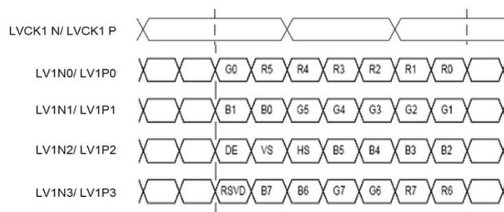
Fig. VESA format
